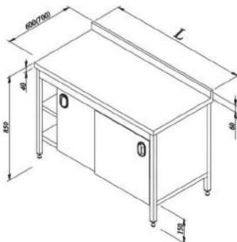
Working Bench With Cupboard Table Adossée Avec Une Étagère Basse Sur Placard
