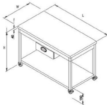
Mobile Bench With Drawer And Shelf Table Centrale Avec Un tiroir Central Et Une Étagère Basse Sur Roulettes
